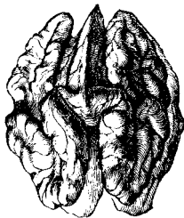
Juglans regia after FAGUET — 1892
